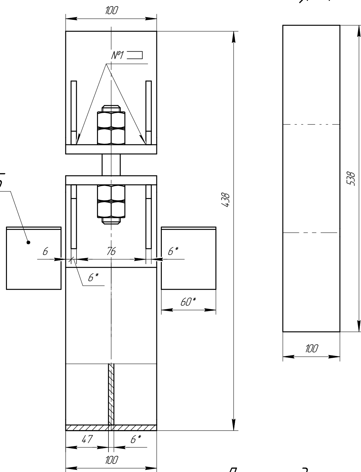
Дет. поз. 3
