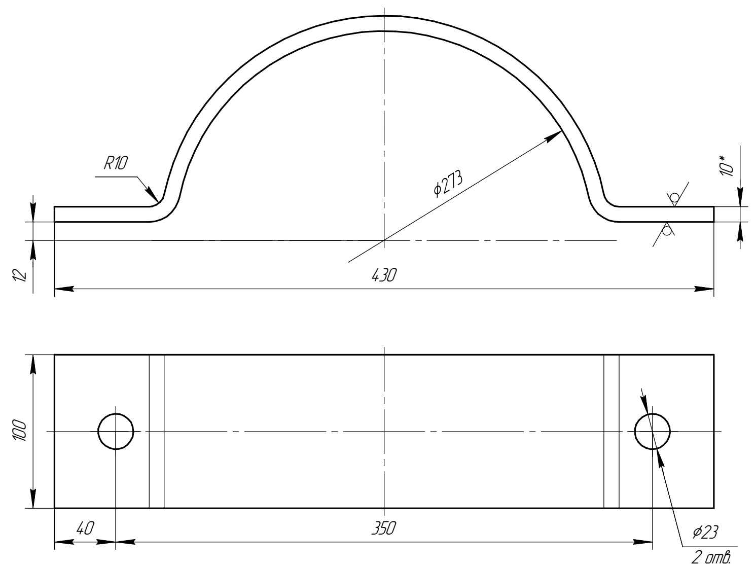
Дет. поз. 2
