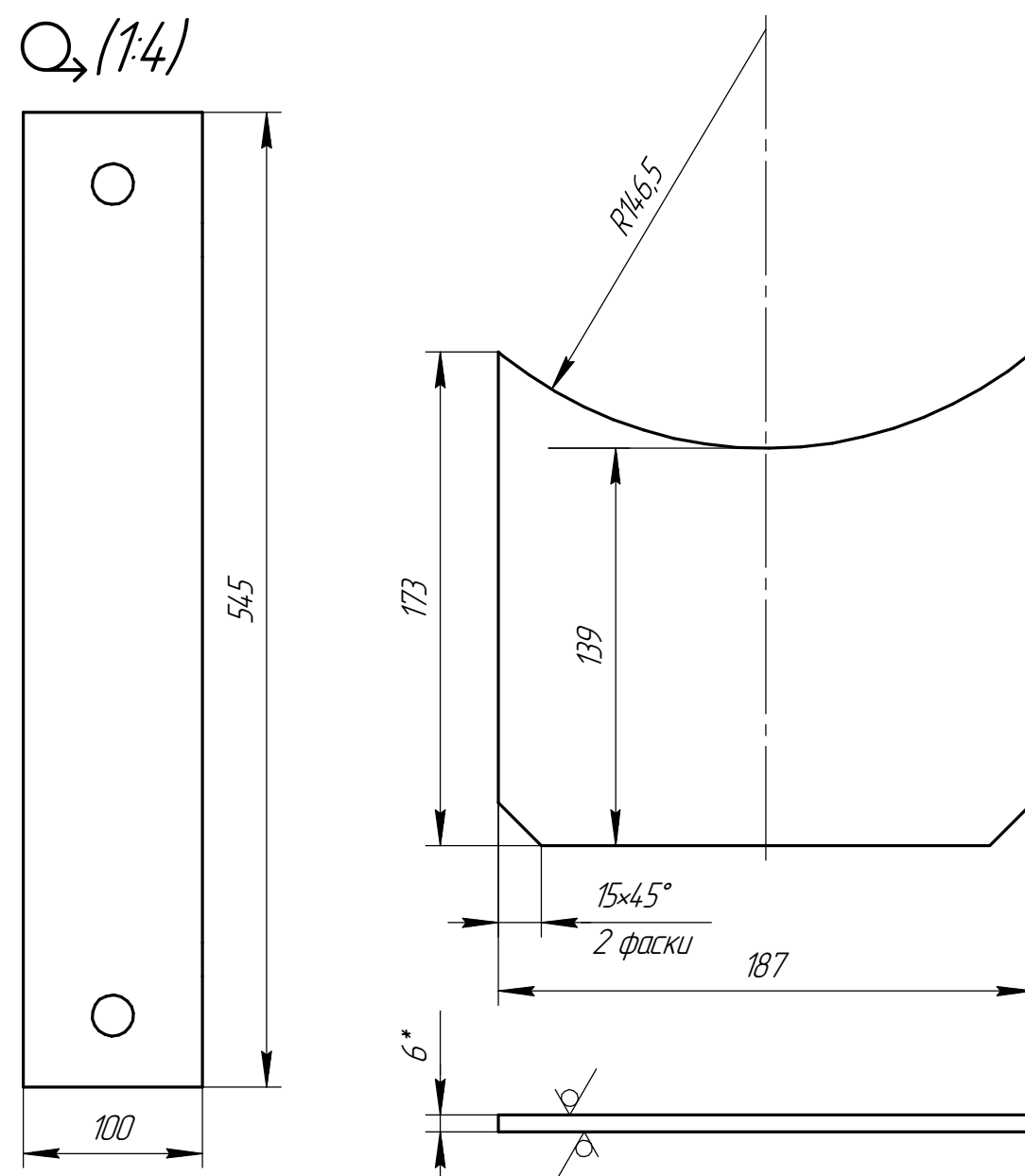
Дет. поз. 3
